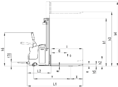
XEH外形图
