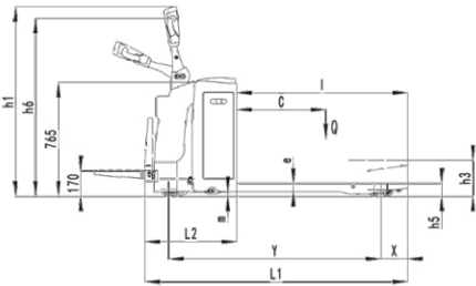
XP20外形图
